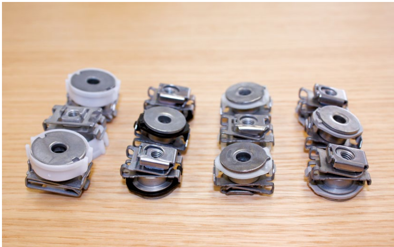
Auswahl bestehender Toleranzausgleichselemente, Produktportfolio Springfix
