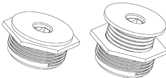
Skizze neues Design, links eingedrehter Zustand, rechts ausgedrehter Zustand
